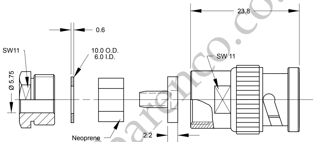
Cable : RG58 - RG223 & Equivalents
